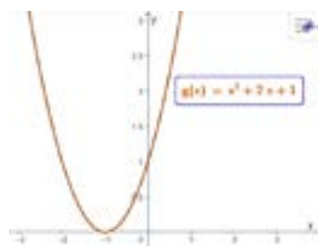
Figura 7. Representación equivalente de la función f(x)
