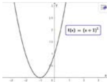
Figura 6. Representación de función cuadrática
